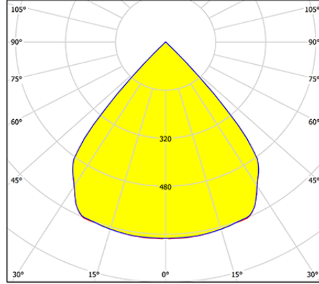
80° - Black Reflector
